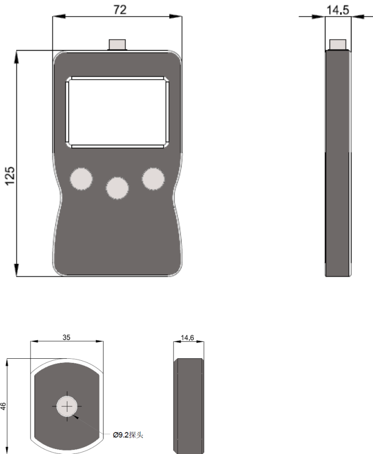
4. FTIU500-365 单波段紫外辐照计外形尺寸:
